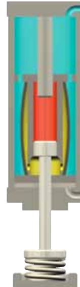
Krafthub mit hydraulischer Druckübersetzung
